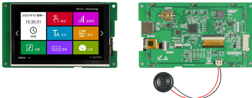
图 1-2 5.0 寸电容触摸参考图
